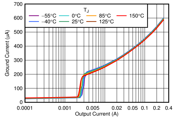
Figure 6-14. I_{\text{GND}} vs I_{\text{OUT}}
